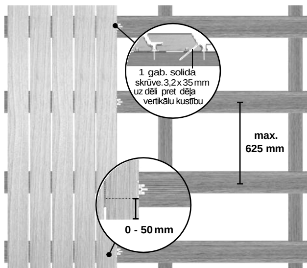
Vertikāla montāža
