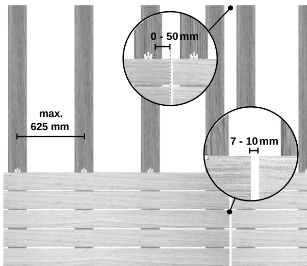
Horizontāla montāža
