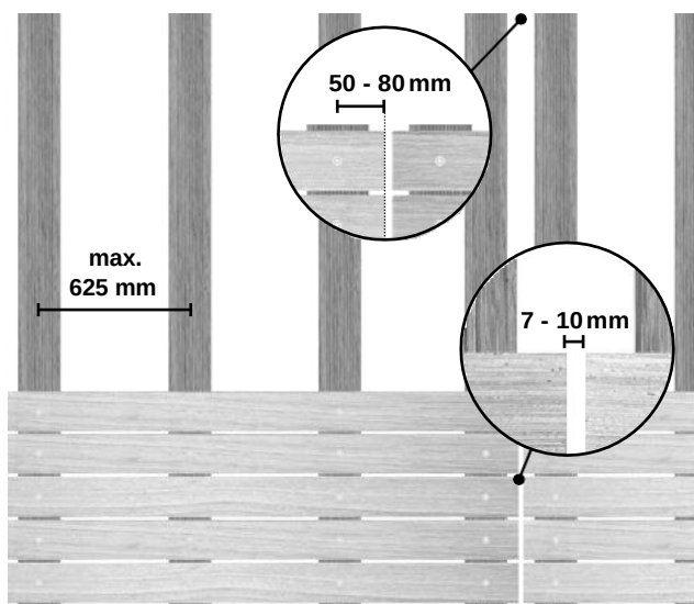
Horizontāla montāža
