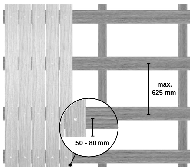
Vertikāla montāža
